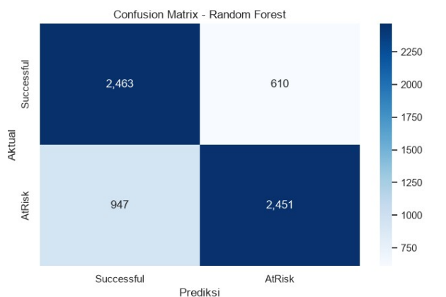
Fig. 4. Confusion matrix Random Forest pada hold-out test.
