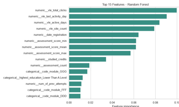
Fig. 6. Lima belas fitur dengan feature importance tertinggi pada Random Forest.
